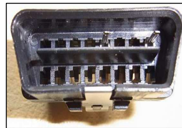
ピン側
