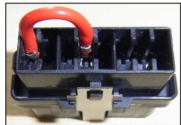
配線側
